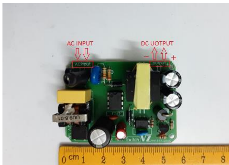
شکل 1: ابعاد آداپتور و مشخص بودن ورودی و خروجی
